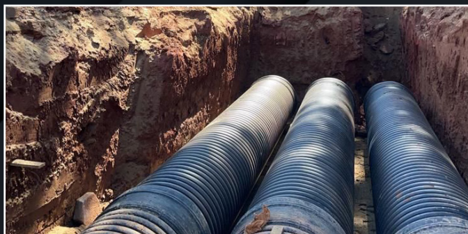
Implantação de rede de drenagem com tubo PEAD envelopado com concreto armado, no município de Pouso Alegre, MG.
