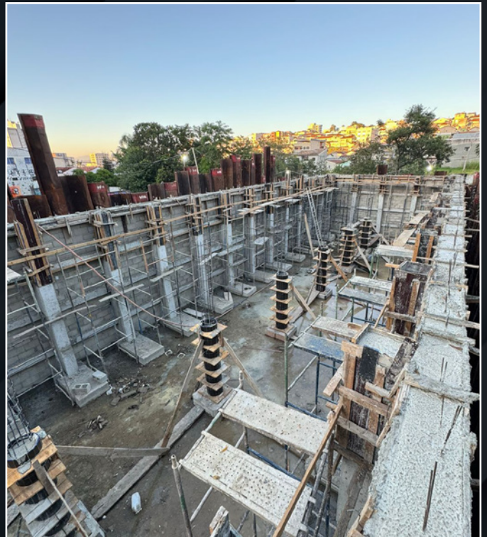
Execução de bacia de retenção de cheias em concreto armado, com capacidade para 1.800,00 m 3 , localizada no município de Pouso Alegre, MG.
